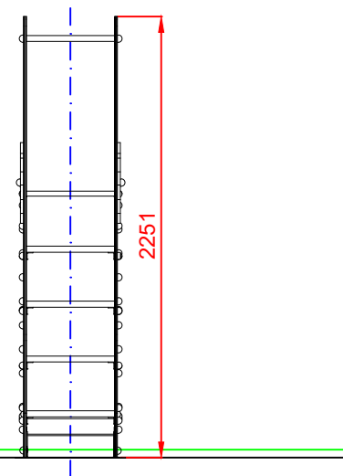
PERFIL IZQUIERDO
