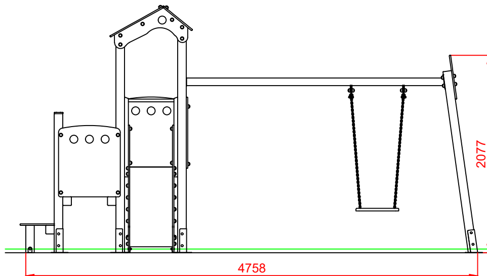
ALZADO
