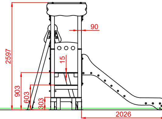
PERFIL IZQUIERDO
