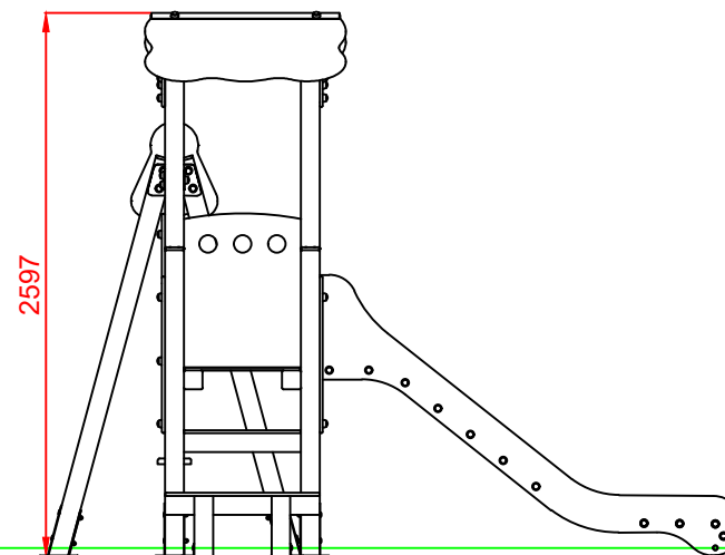
PERFIL IZQUIERDO
