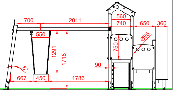
ALZADO POSTERIOR
