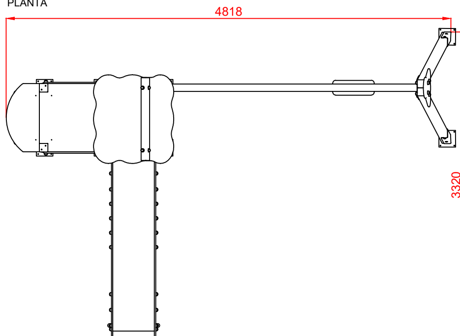
PLANTA
