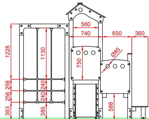
PERFIL IZQUIERDO
