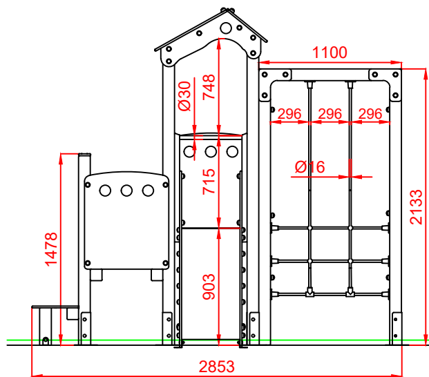
PERFIL DERECHO
