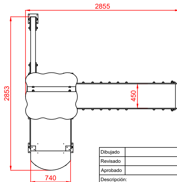
PLANTA
