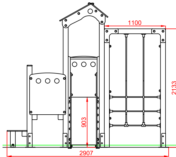
PERFIL DERECHO
