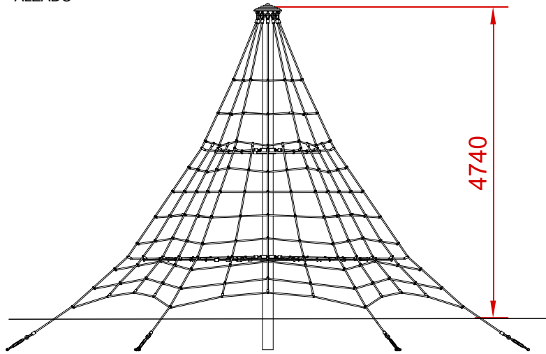
ALZADO
