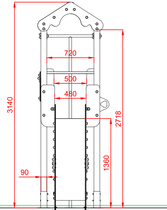
PERFIL IZQUIERDO
