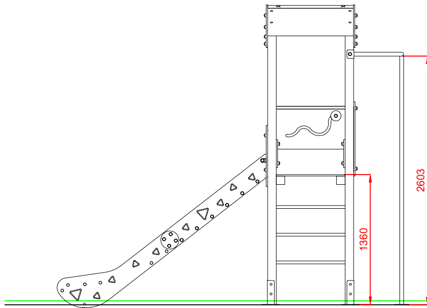
ALZADO
