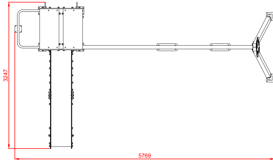
PLANTA
