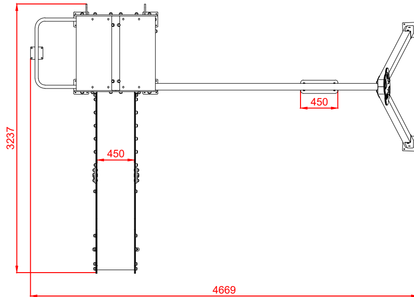
PLANTA
