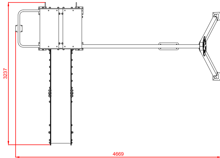
PLANTA
