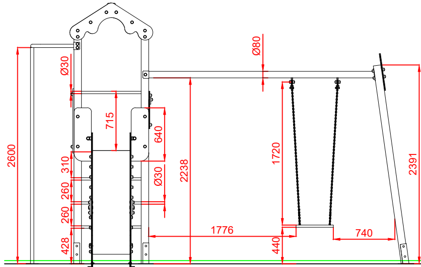
ALZADO
