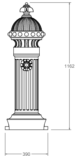
vista frontal 1:20
