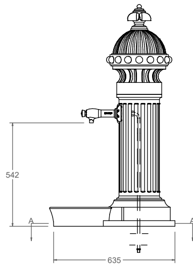
vista alzado 1:20
