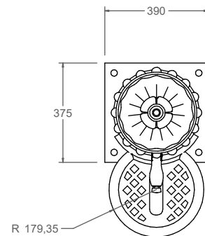
vista en planta 1:20
