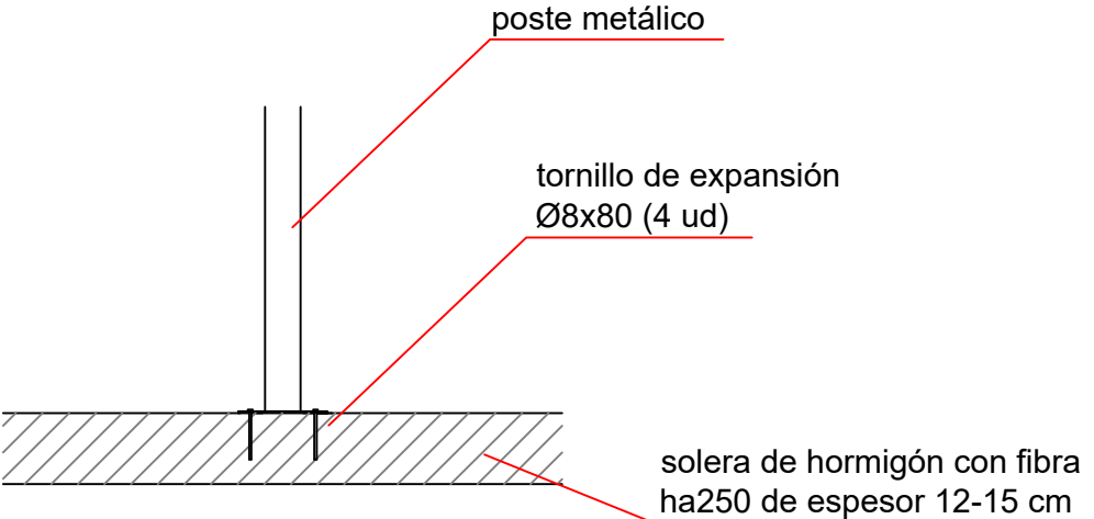
DETALLE DE ANCLAJE
