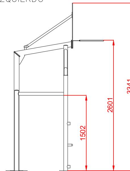
PERFIL IZQUIERDO
