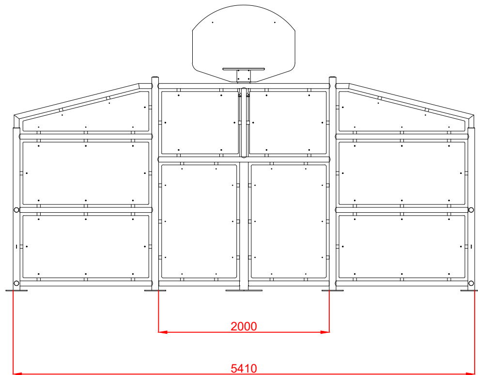
ALZADO
