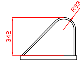
Vista Perfil
