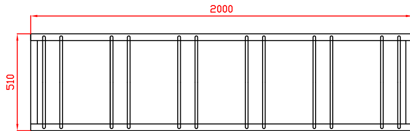
Vista Planta
