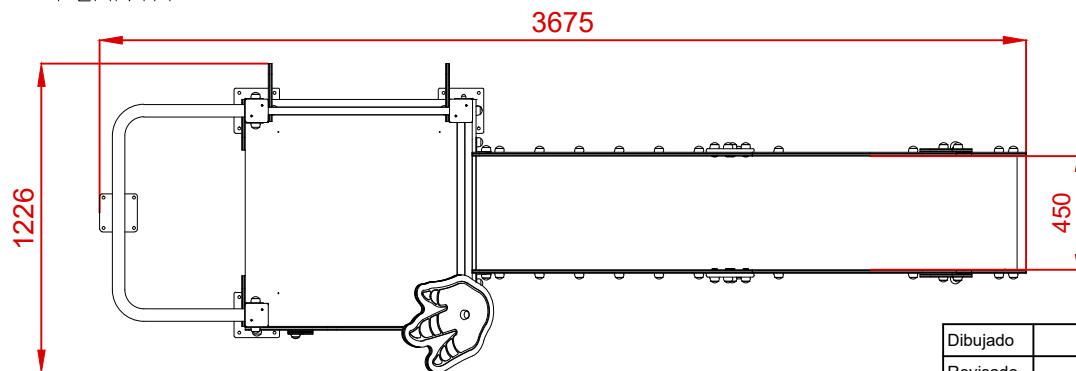
PLANTA
