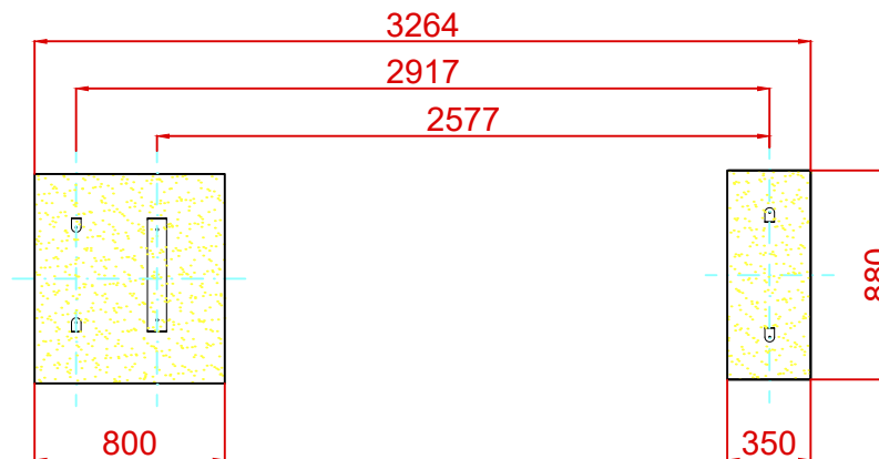
PLANTA CIMENTACIÓN
