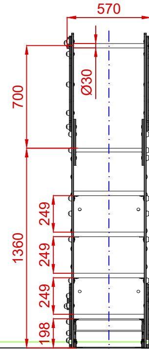
PERFIL
