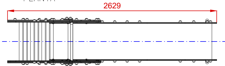
PLANTA
