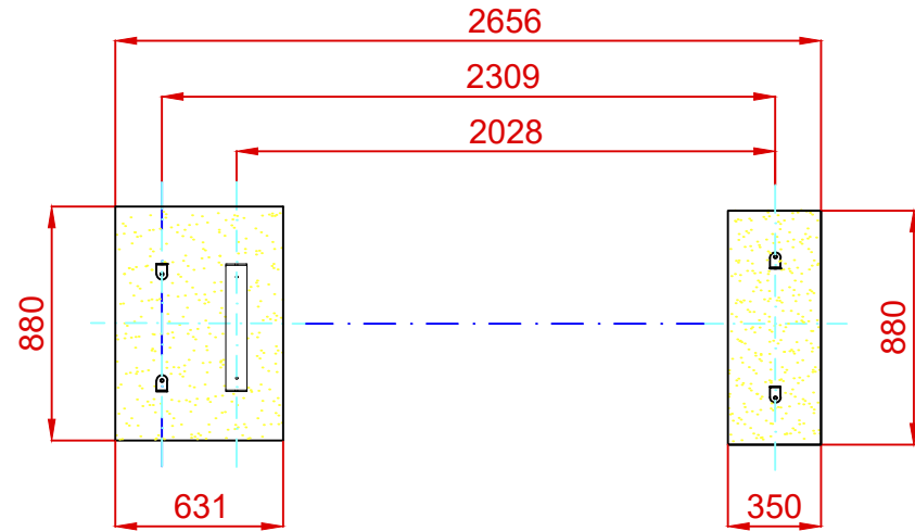
PLANTA CIMENTACIÓN
