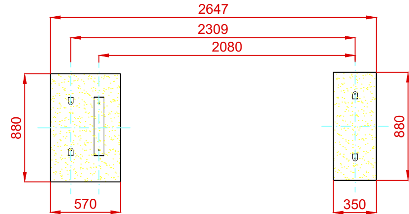
PLANTA CIMENTACIÓN
